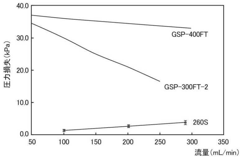
260Sの流量と圧力損失の関係
